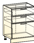
Монако шкаф рабочий (3 ящика) → | 7 | ↑ 600|460|820
