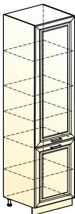
Атланта шкаф-пенал 2 (2 двери) → | 7 | 1 | ↑ 600|570|2141
