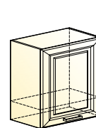
Атланта шкаф навесной под вытяжку (1 дверь глухая) → | 7 | ↑ 600|318|566
