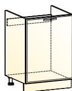
Монако шкаф рабочий под мойку (1 дверь) → | 7 | ↑ 600|456|820
