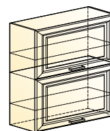
Атланта шкаф навесной (2 двери горизонт.) → | 7 | ↑ 800|318|900
