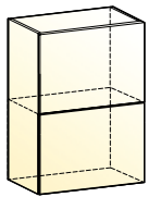
Бостон шкаф навесной (2 двери горизонт.) → | 7 | 1 | ↑ 500|318|720
