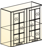
Бавария шкаф навесной (2 двери рамочные) → | 71 | ↑ 800|318|720
