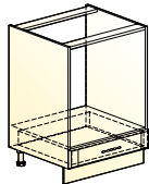
Бавария шкаф рабочий под духовку (1 ящик) → | 1 | 1 | ↑ 600|460|820
