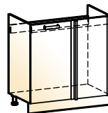
Яна шкаф рабочий под мойку угловой (1 дверь) → | 7 | ↑ 800|486|820
