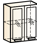
Яна шкаф навесной (2 двери рамочный) → | ↑ | ↑ 600|318|720
