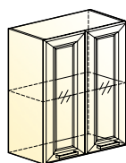
Атланта шкаф навесной (2 двери рамочный) → | 7 | ↑ 600|318|720
