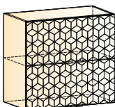
Стоун шкаф навесной (2 двери горизонт. с фрез.) → | 7 | 1 | ↑ 800|318|720
