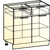
Бостон шкаф рабочий (2 двери 2 ящика) → | 7 | 1 | ↑ 800|460|820
