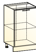
Монако шкаф рабочий (1 дверь) → | 7 | ↑ 500|460|820
