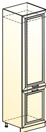
Атланта шкаф-пенал под холодильник (2 двери) → | 7 | 1 | ↑ 600|570|2141
