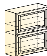
Мишель шкаф навесной (2 двери горизонт.) → | 7 | ↑ 800|318|900
