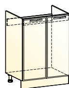
Монако шкаф рабочий под мойку (2 двери) → | 7 | ↑ 600|456|820
