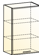
Монако шкаф навесной (1 дверь глухая) → | 7 | 1 | ↑ 600|318|900
