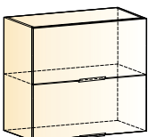
Стоун шкаф навесной (2 двери горизонт.) → | 7 | 1 | ↑ 800|318|720
