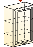
Атланта шкаф навесной (1 дверь глухая) → | 7 | ↑ 600|318|900
