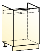
Стоун шкаф рабочий под мойку (1 дверь) → | 7 | ↑ 600|456|820
