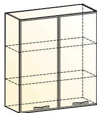
Монако шкаф навесной (2 двери глухие) → | 7 | 1 | ↑ 800|318|900
