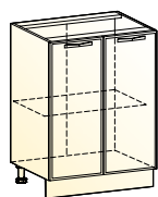
Монако шкаф рабочий (2 двери) → | 7 | ↑ 600|460|820
