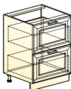
Атланта шкаф рабочий (2 ящика) → | 1 | 1 | ↑ 600|460|820
