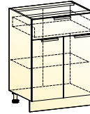
Бостон шкаф рабочий (2 двери 1 ящик) → | 7 | 1 | ↑ 600|460|820
