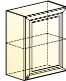
Мишель шкаф навесной (1 дверь глухая) → | 7 | 1 | ↑ 600|318|720
