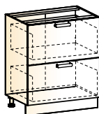
Яна шкаф рабочий (2 ящика) → | 7 | ↑ 800|460|820
