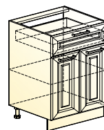
Мишель шкаф рабочий (2 двери 1 ящик) → | 7 | ↑ 600|460|820
