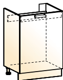
Яна шкаф рабочий под мойку (1 дверь) → | 7 | ↑ 600|456|820
