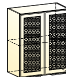
Стоун шкаф навесной (2 двери рамочный) → | 7 | 1 | ↑ 600|318|720
