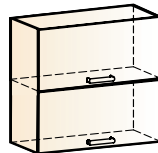
Яна шкаф навесной (2 двери горизонт.) → | ↑ | ↑ 800|318|720
