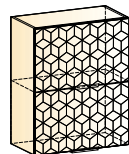
Стоун шкаф навесной (2 двери горизонт. с фрез.) → | 7 | 1 | ↑ 600|318|720
