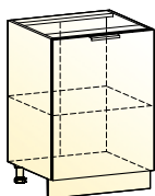
Стоун шкаф рабочий (1 дверь) → | 7 | ↑ 600|460|820
