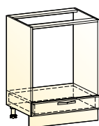
Монако шкаф рабочий под духовку (1 ящик) → | 7 | ↑ 600|460|820
