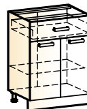
Яна шкаф рабочий (2 двери 1 ящик) → | 7 | ↑ 600|460|820
