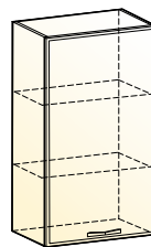
Монако шкаф навесной (1 дверь глухая) → | 7 | 1 | ↑ 500|318|900
