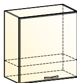
Монако шкаф навесной под вытяжку (1 дверь глухая) → | 7 | | ↑ 600|318|566
