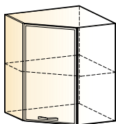
Монако шкаф навесной угловой (1 дверь глухая) → | 7 | | ↑ 600|600|720
