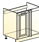
Атланта шкаф рабочий под мойку угловой (1 дверь) → | 1 | 1 | ↑ 800|486|820
