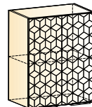
Стоун шкаф навесной (2 двери глухие с фрез.) → | 7 | 1 | ↑ 600|318|720
