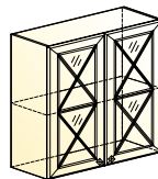
Мишель шкаф навесной (2 двери крестовина) → | 7 | 1 | ↑ 800|318|720
