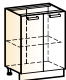
Яна шкаф рабочий (2 двери) → | 7 | ↑ 600|460|820
