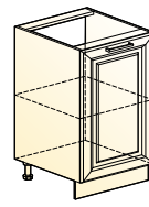
Мишель шкаф рабочий (1 дверь) → | 7 | ↑ 450|460|820
