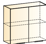
Стоун шкаф навесной (2 двери глухие) → | 7 | 1 | ↑ 800|318|720
