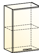
Монако шкаф навесной (1 дверь глухая) → | 7 | | ↑ 500|318|720
