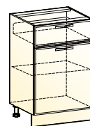
Монако шкаф рабочий (1 дверь 1 ящик) → | 7 | ↑ 500|460|820
