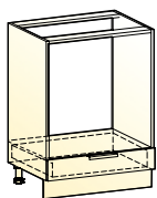
Стоун шкаф рабочий под духовку (1 ящик) → | 7 | ↑ 600|460|820
