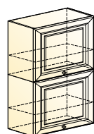
Мишель шкаф навесной (2 двери горизонт.) → | 7 | ↑ 600|318|900
