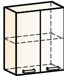
Яна шкаф навесной (2 двери глухие) → | ↑ | ↑ 600|318|720
